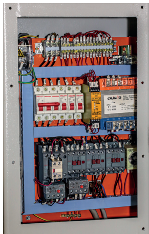
Três micros de segurança que consta na estrutura da mesma para segurança do operador e mantenedor
