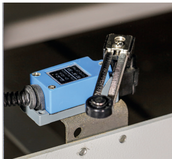
Micro N° 2 ao abrir a máquina para manutenção para troca do motor principal, limpeza e manutenção na porta de acesso tem uma micro, ao abrir a porta a mesma ira atuar desligando toda máquina informando para o operador que a mesma não entrar em operação
