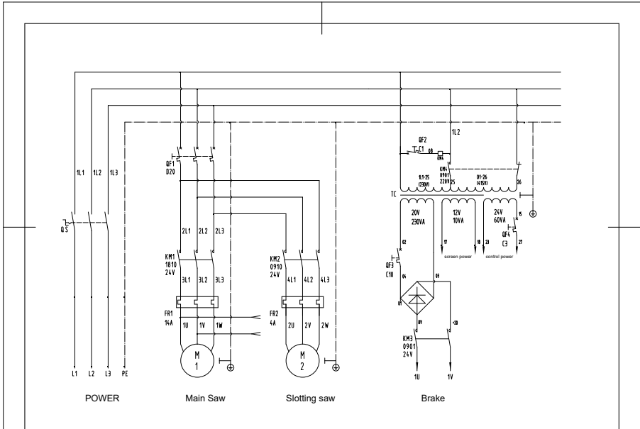
青岛永强 设备名称: 精密裁板锯 型号: MJ- 制图: 日期: 2020-12-27 第页: 01 共页: 03
